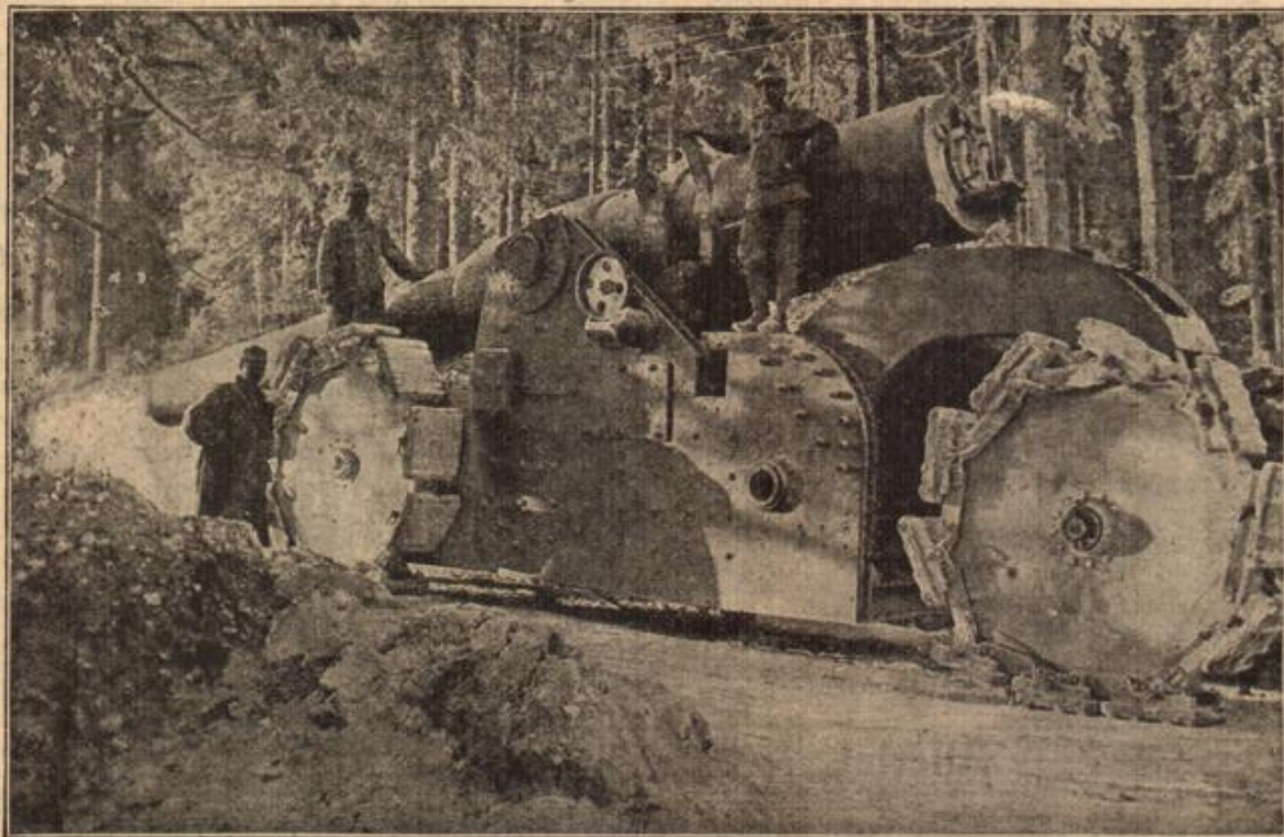
Ein erobertes italienisches Schiffsgeschütz, das in den österreichisch-ungarischen Stellungen gegen seine früheren Besitzer verwandt wird.
