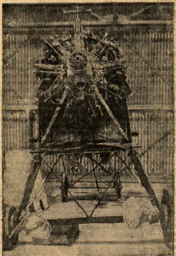
Zum Kampf in den Lüften: Der Motor eines erbeuteten Loisin-Flugzeuges.
