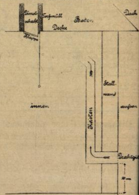
Künstliche Lüftungsanlage.
