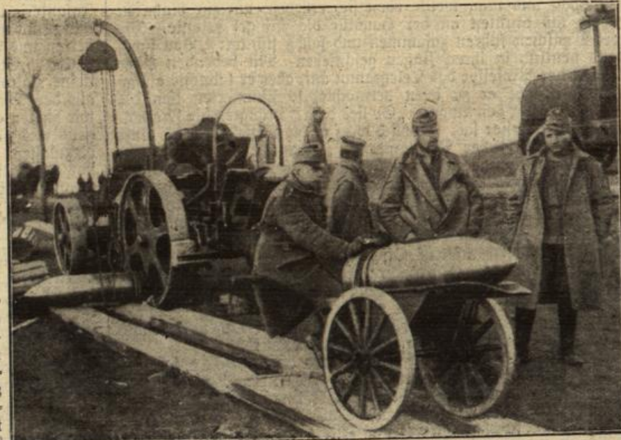
Geschloßwagen der österr. 30,5 cm-Motormörser mit einem Gesch. (Mit Text.)
