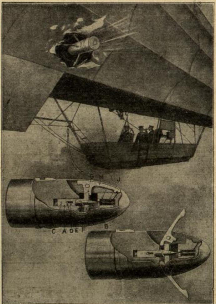
Explosionsgeschloß zur Vernichtung von Luftschiffen. (Mit Text.)
