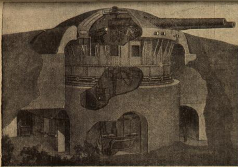
Turfschnitt durch einen französischen Panzerturm.
