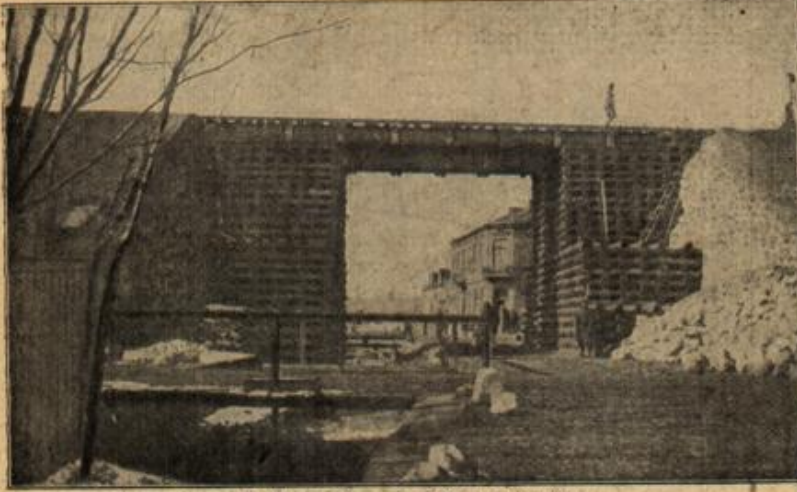
Notbrückenbau aus Bahnschwellen.
