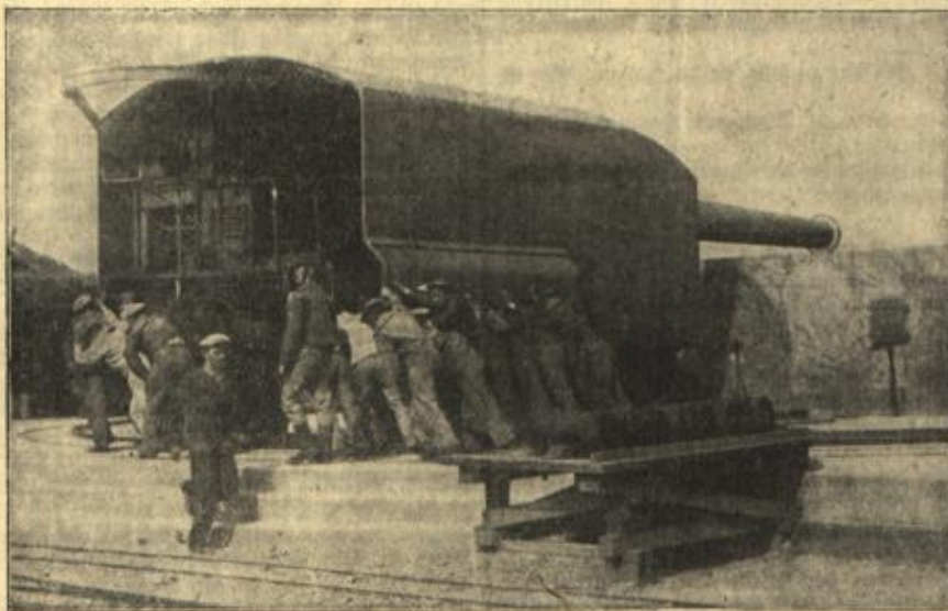
Vom Schutz der flandrischen Küste: Geschützdröhen in einer deutschen Küstenbatterie.
