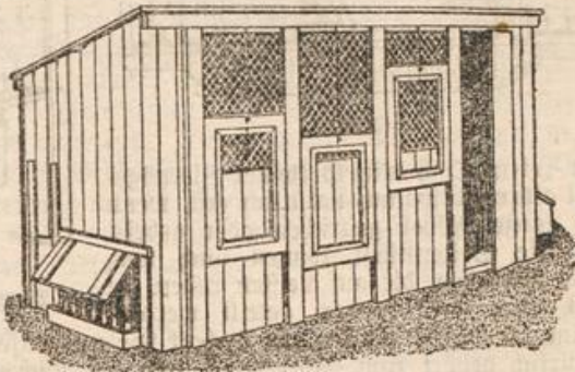
Abb. 2. Hühnerhaus mit Scharraum, 3,5 m lang, 2 m tief, 2,50 m hoch, links Futtertrog, rechts Schlafraum mit außen seitigen Regenestern.
